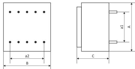
TEZ 0,5 - 16
