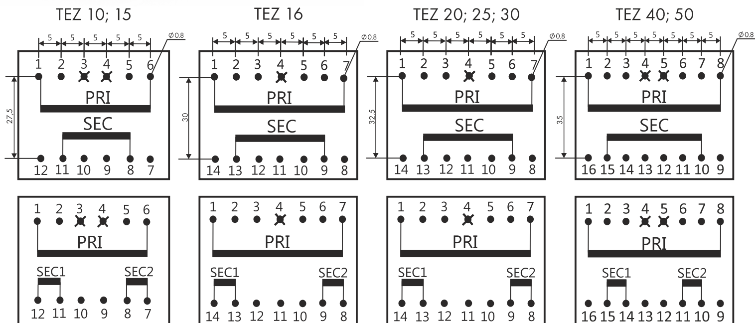
Beispiel zur Identifizierung der Pinbelegung auf der Grundlage von TEZ 10.
